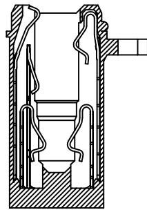
SECTION:B-B
